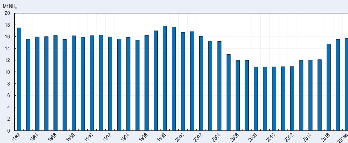
Graphique 1.10. Capacité de production d'ammoniac des États-Unis
