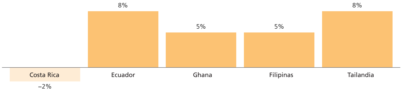
Figura 6. Porcentaje de cambio de precipitación para 2100 utilizando el modelo SSP2-4.5, en países productores de piña
