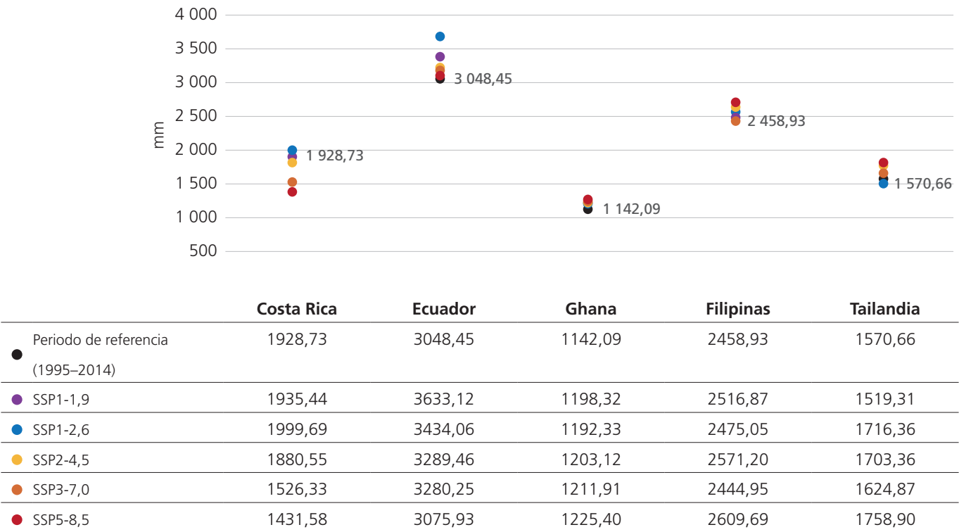
Figura 5. Precipitación media proyectada para 2100, período de referencia 1995–2014, para los países productores de piña
