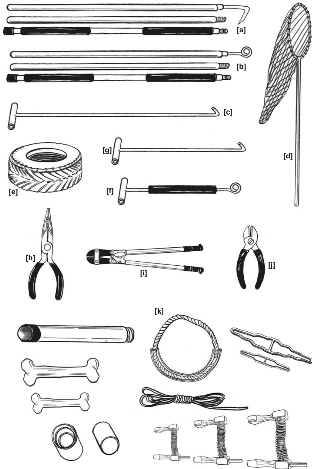
Figure 26. Matériel utilisé pour manipuler et remettre en liberté les tortues de mer. Selon le Service des pêches nord-américain (United States National Marine Fisheries Service) cet équipement est obligatoire à bord des palangriers nord-américains qui opèrent dans l'Atlantique (d'après le US National Marine Fisheries Service, 2004).
