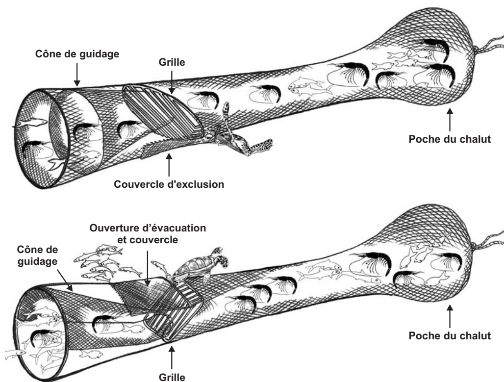
Figure 16. Différents éléments normalement intégrés dans un DET à exclusion par le bas et un DET à exclusion par le haut.
