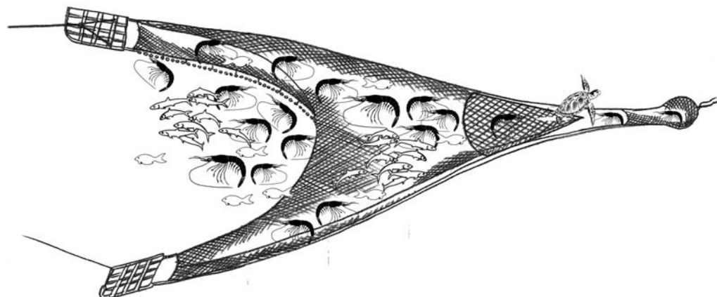
Figure 18. Le DET Morrison, un exemple de DET souple (d'après Eayrs, 2007)
