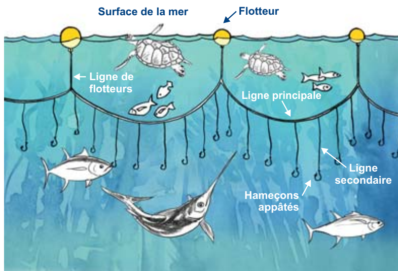
Figure 8b. Une ligne de flotteurs plus courte diminue la profondeur de mouillage
