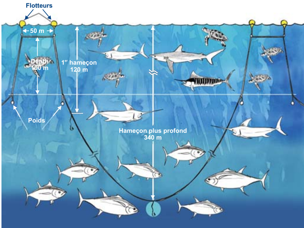
Figure 15. Configuration de lignes lestées avec 20 hameçons par panier et une profondeur cible pour les hameçons les moins profonds de 120 m. Des exemples d'espèces cibles et accessoires possibles sont présentés: à moins de 100 m, il s'agit notamment de tortues de mer, de requins et de marlins, tandis qu'à plus de 100 m, le thon obèse et l'espadon sont capturés. Tous les hameçons appâtés se trouvent à plus de 100 m de profondeur (d'après Beverly et Robinson, 2004).
