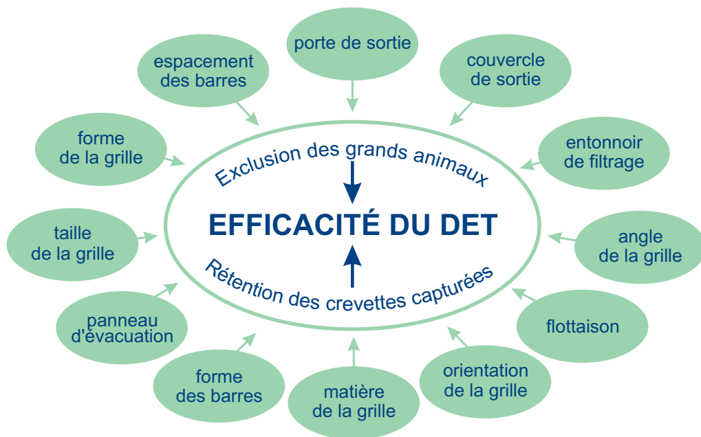
Figure 19. Facteurs influençant l'efficacité des DET
