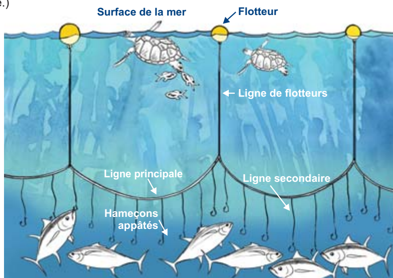
Figure 8a. Une ligne de flotteurs plus longue augmente la profondeur de mouillage
